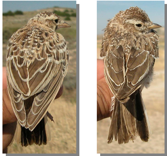
Diseño del dorso: izquierda torrera común; derecha torrera marismeña.
