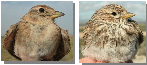
Diseño del pecho: izquierda torrera común; derecha torrera marismeña.
